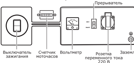
УГБ-2000, УГБ-2500, УГБ-3200, УГБ-3200Е
