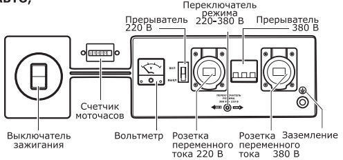
Трехфазный генератор: УГБ-6000ЕТ/380В, УГБ-6700ЕТ/ 380 В, УГБ-7500ЕТ/ 380 В, УГБ-8200ЕТ/380 В
